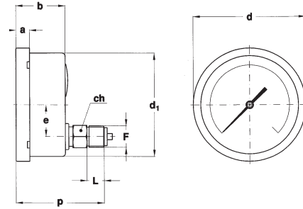
D - POSTERIOR para montaje local directo
